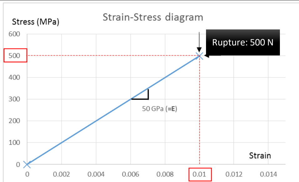
Fig 1b4.3 | Diagramme contrainte – déformation relative du matériau
